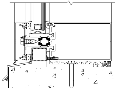
④ Sill
