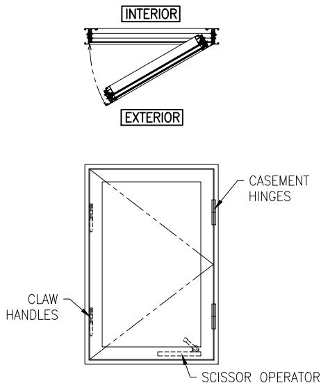
CASEMENT WINDOW OPEN-OUT (S.H.O.O.)
