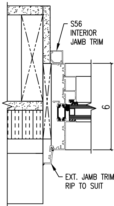
JAMB
